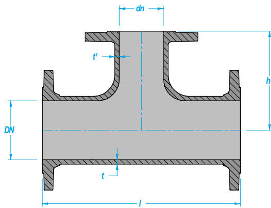
FIG. 1 TEES FLG/FLG/FLG
