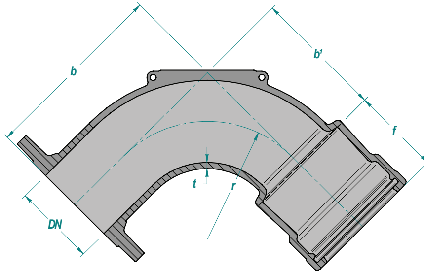
Bend FLG/SOC 90°
